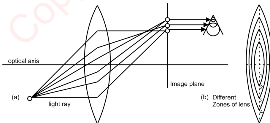
Fig. 2.6 Coma
