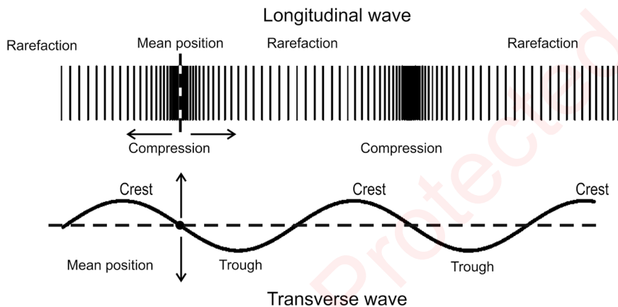
Fig. 1.4 Longitudinal and transverse waves
